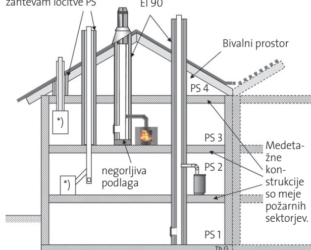
Risba 17: Zahteve za dimnovodne naprave pri horizontalni delitvi na požarne sektorje pri kurilnih napravah na trda goriva, olje ali plin
