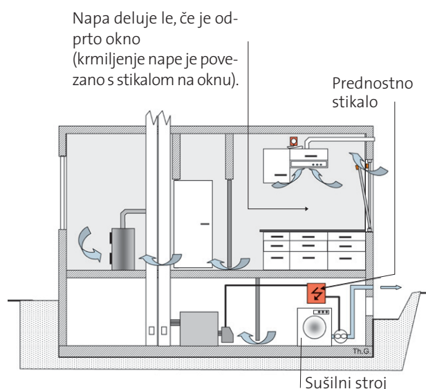
Risba 5: Zagotavljanje varnosti obratovanja z izpolnjevanjem pogoja iz prve in druge alinee drugega (2) odstavka točke 4
