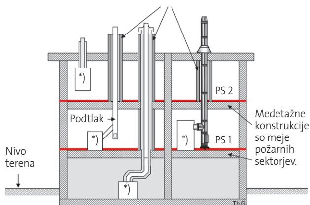
Risba 16: Zahteve za dimnovodne naprave pri horizontalni delitvi na požarne sektorje pri kurilnih napravah na olje ali plin
