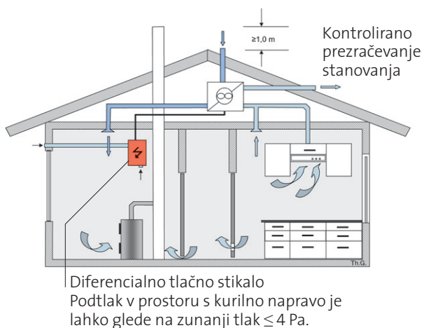
Risba 6: Zagotavljanje varnosti obratovanja z izpolnjevanjem pogoja iz prve in druge alinee drugega (2) odstavka točke 4
