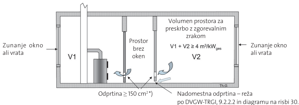
Risba 1: Zagotavljanje zgorevalnega zraka po prvi alineji prvega (1) odstavka točke 3
