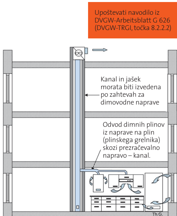
Risba 7: Zagotavljanje varnosti obratovanja z izpolnjevanjem pogoja iz druge in četrte alinee drugega (2) odstavka točke 4
