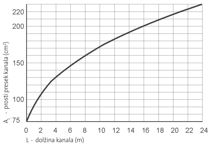
Risba 28: Izračun ekvivalentnega preseka kanala A_L glede na dolžino kanala L , ki ustreza zahtevi po prostem preseku odprtine za dovod zraka 150 cm²
